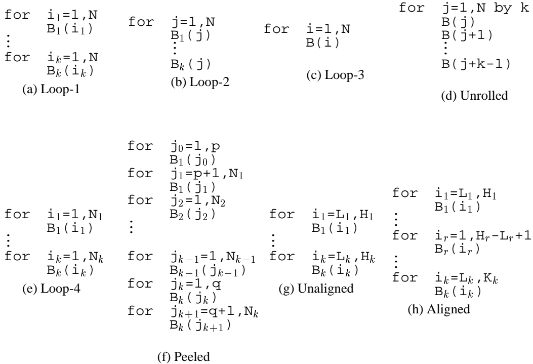
Fig. 4. Loop Transformations
